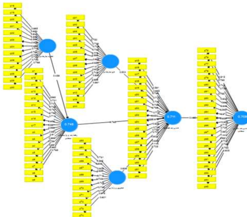
Fig 3: R 2 Values
